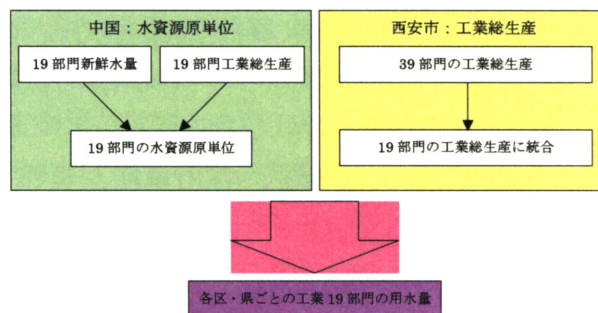
図-2 工業用水推計フロー
