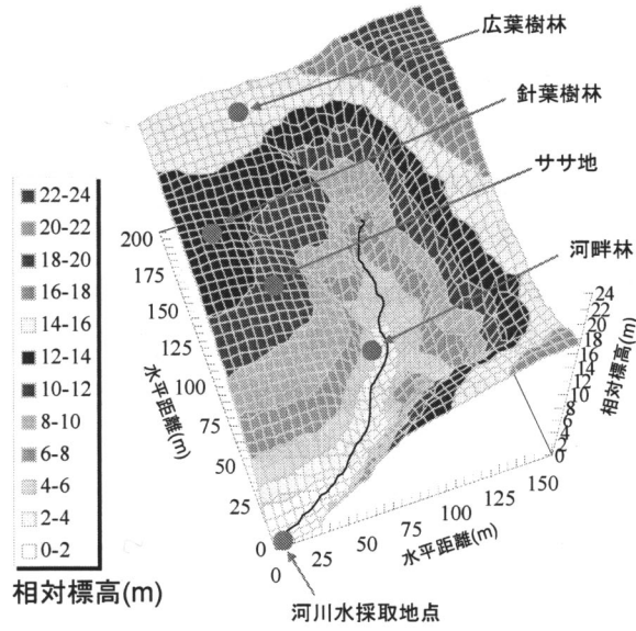
図 1. 流域内における土壌溶液と河川水採取地点の位置図
