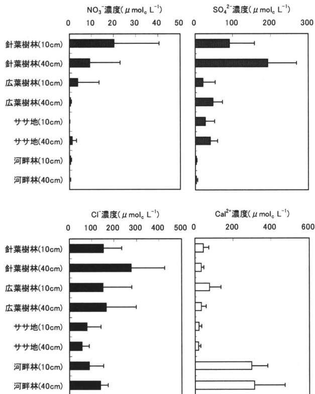
図 2. 各林分における土壌溶液(10cm, 40cm)のイオン濃度(2006年7~9月の平均値)
